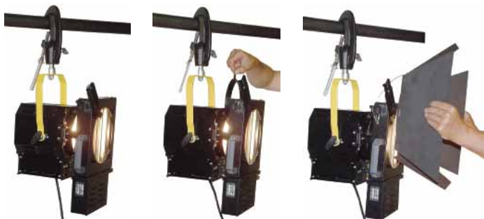
灯体前面部のランナーに JALOUSIE ②を取付ます / Place the JALOUSIE ② in the front runner. 次のランナーにライトシールドを取付ます / Place the light shield in the next runner. ブラインドの全面にバンドアを取付ます / Place the barndoor at the front of the JALOUSIE ②.
